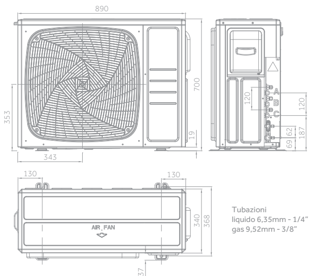
5U90S2SS2FA (5 attacchi)
