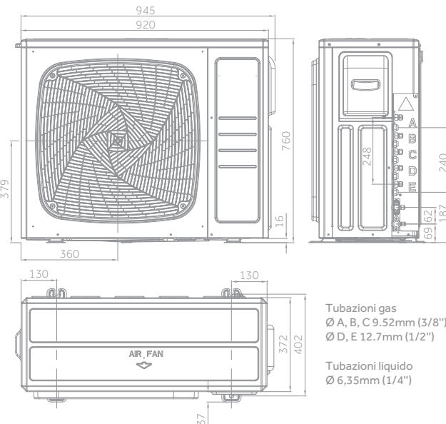
5U105S2SS3FA (5 attacchi)
