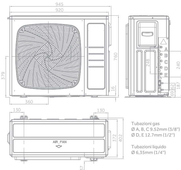
5U90S2SS2FA (5 attacchi)
